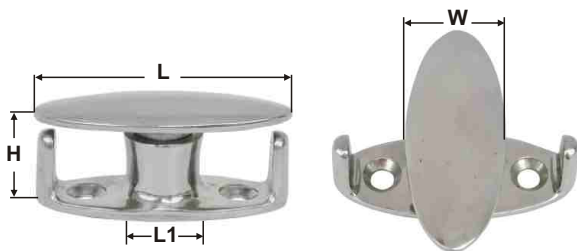
FENDER HALTER MIT DREHVERSCHLUSS AISI 316
